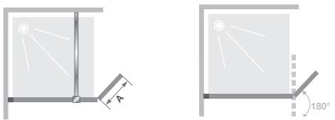
Volet pivotant installé avec la paroi Smart Design Solo
