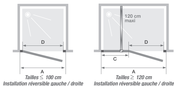
Smart Express P sans seuil (taille ≤ 100 cm) - profilé chromé - verre transparent
