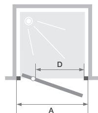
Tailles ≤ 100 cm Installation réversible gauche / droite
