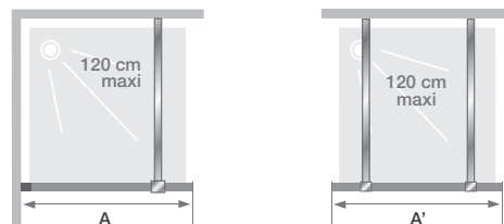
Installation réversible gauche / droite
