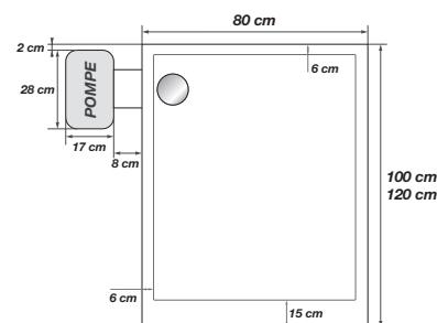
pompe à gauche
