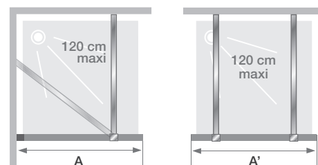
Installation réversible gauche / droite
