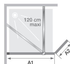
Ouverture du volet pivotant à 180°
