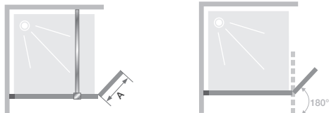
Volet pivotant installé avec la paroi Smart Design Solo
