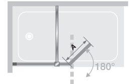
Combinaison Smart Design Hydra + volet pivotant
